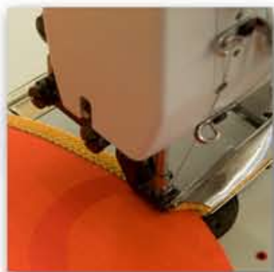
La piegatura del bordino avviene in prossimità dell'ago. In questa maniera si possono bordare senza problemi anche raggi minimi.
